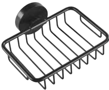
■ Tvålkorg Soap basket | Seifenhalter 140 x 55 x 125 mm 104108160
